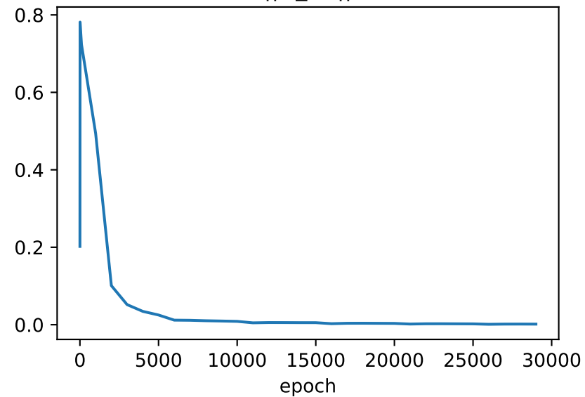
||H_{dir}||
