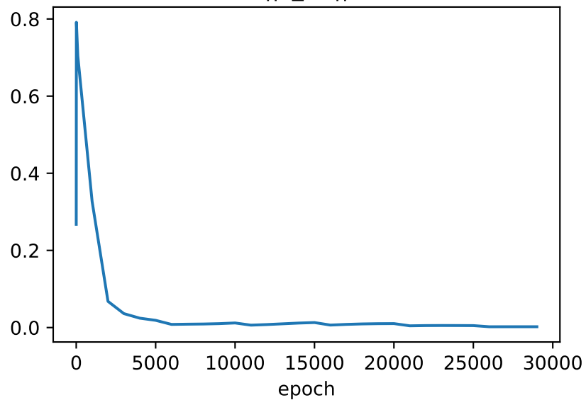
||L_{dir}||
