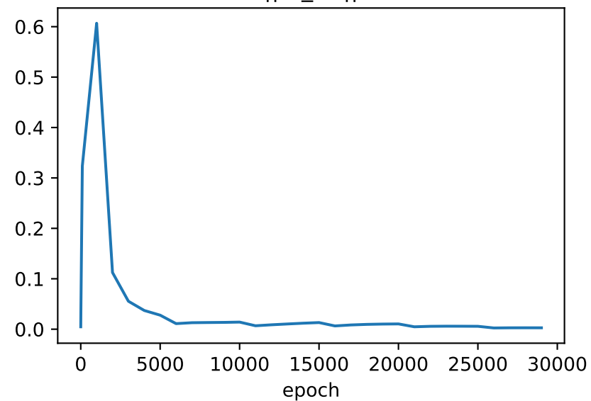
||W_{dir}||
